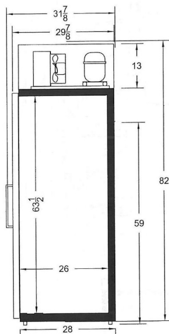
Modèle FSH48T (Compresseur en haut)
